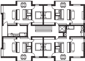
A1 tipična etaža
