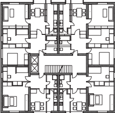
B3 tipična etaža
