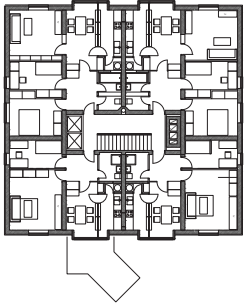
B2 tipična etaža
