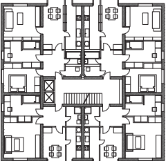
B1 tipična etaža
