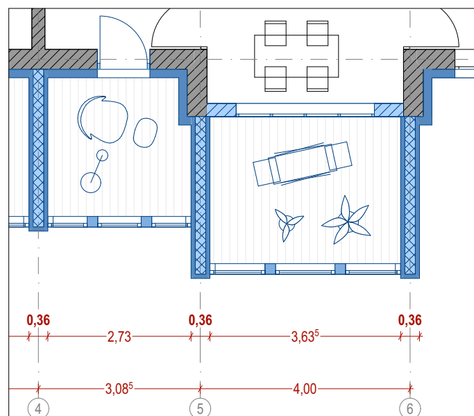
VARIANTA 1: BETONSKA REBRA + STEBRIČI
